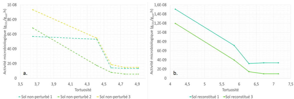
Figure 1: Variation de l'activité microbologique et de la tortuosité en fonction de la conductivité électrique pour (a) les échantillons non-perturbés et (b) les échantillons reconstitués. Chaque point correspond à une saturation différente (d'après Bouakkaz, 2018).
